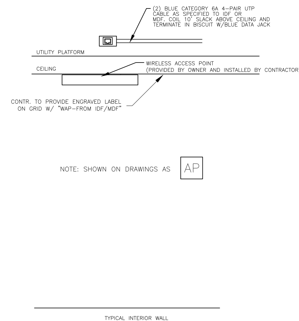
001.5 WAP OUTLET DETAIL SCALE: NONE
