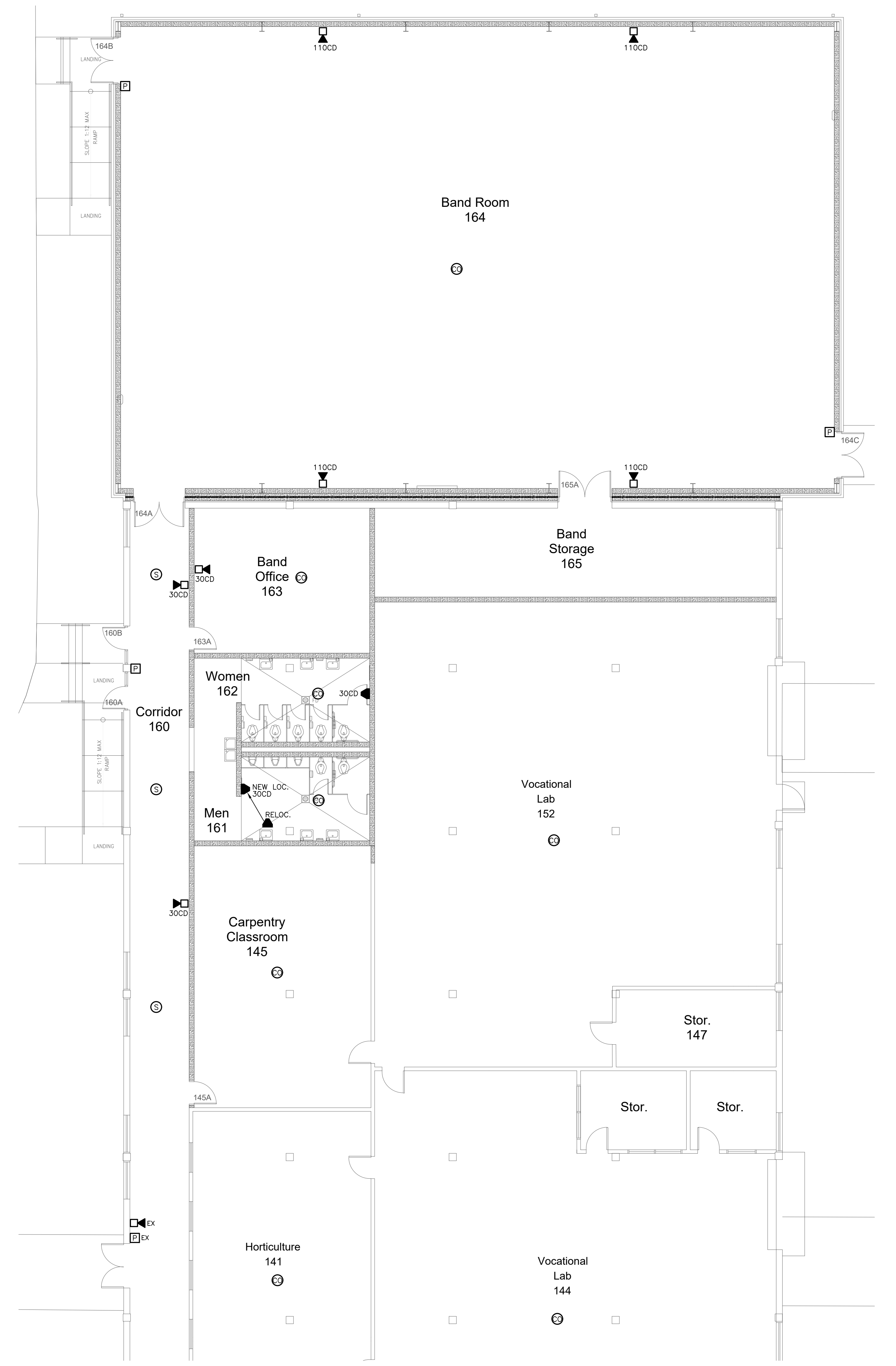
111.1 BAND RM ADD'N FIRE ALARM PLAN SCALE: 1/8" = 1'-0"
